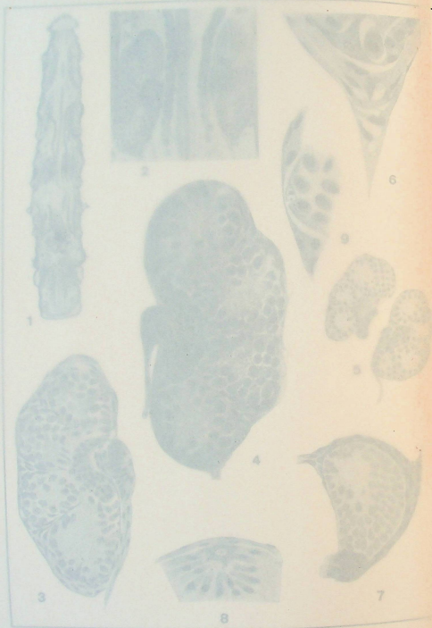
Fig. 1-8. - Ghiandole parietali...
