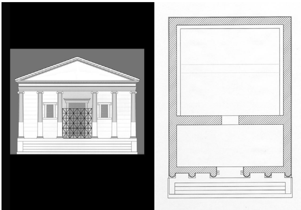
Fig. 5. Gortina, pianta e ricostruzione del prospetto del Tempio (da LIPPOLIS - LIVADIOTTI - ROCCO 2005).
